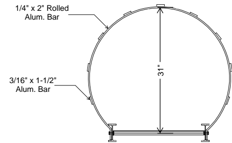
(D) Bottom Hoop Detail
